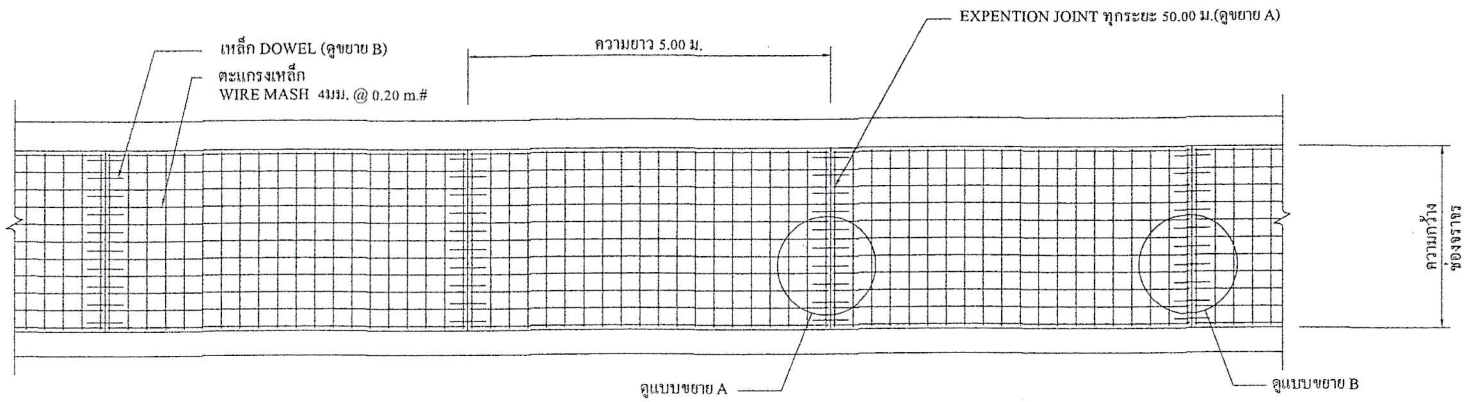
แปลนแสดงการเสริมเหล็กถนน SCALE noscale
