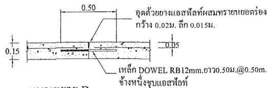
แบบขยชย B SCALE noscale
