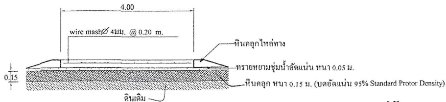
รูปตัดตามขวางผิวจราจร SCALE noscale
